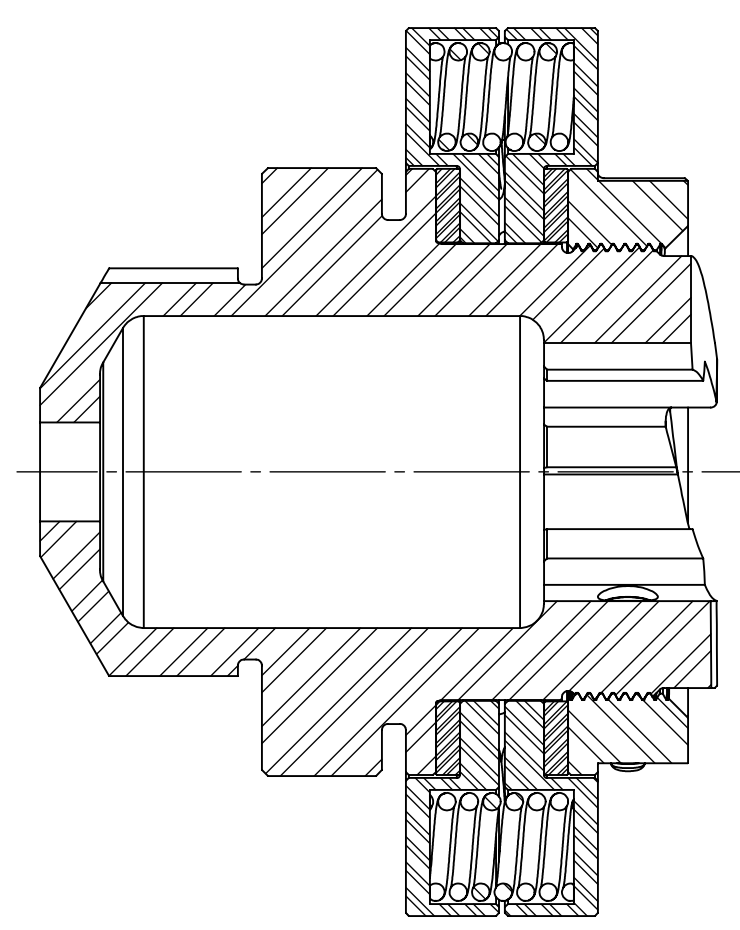
SECTION A-A
